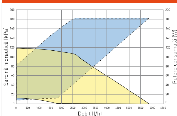
Grafic debit/sarcină hidraulică VICTRIX PRO 120 ErP
