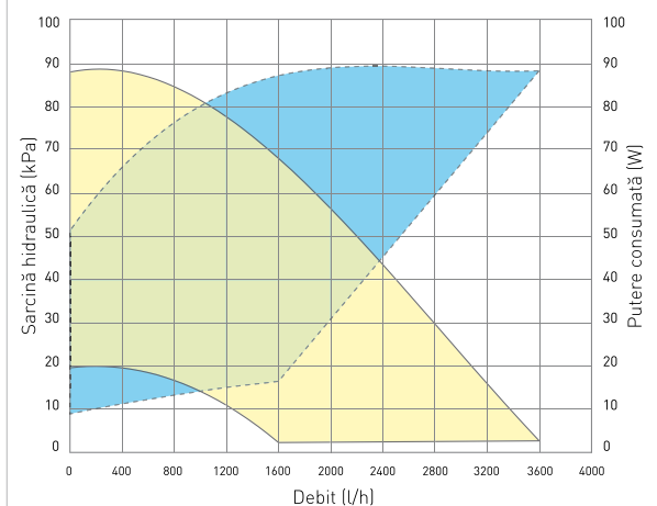
Grafic debit/sarcină hidraulică VICTRIX PRO 80 ErP
