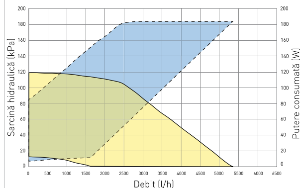
Grafic debit/sarcină hidraulică VICTRIX PRO 100 ErP
